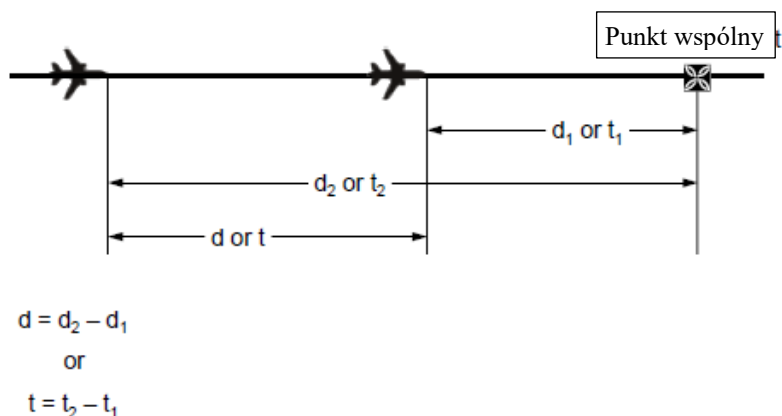
Rysunek 5-30. Obliczanie odległości podłużnej / czasu między statkami powietrznymi – identyczna linia drogi, ten sam kierunek (patrz 5.4.2.9.5 a))
