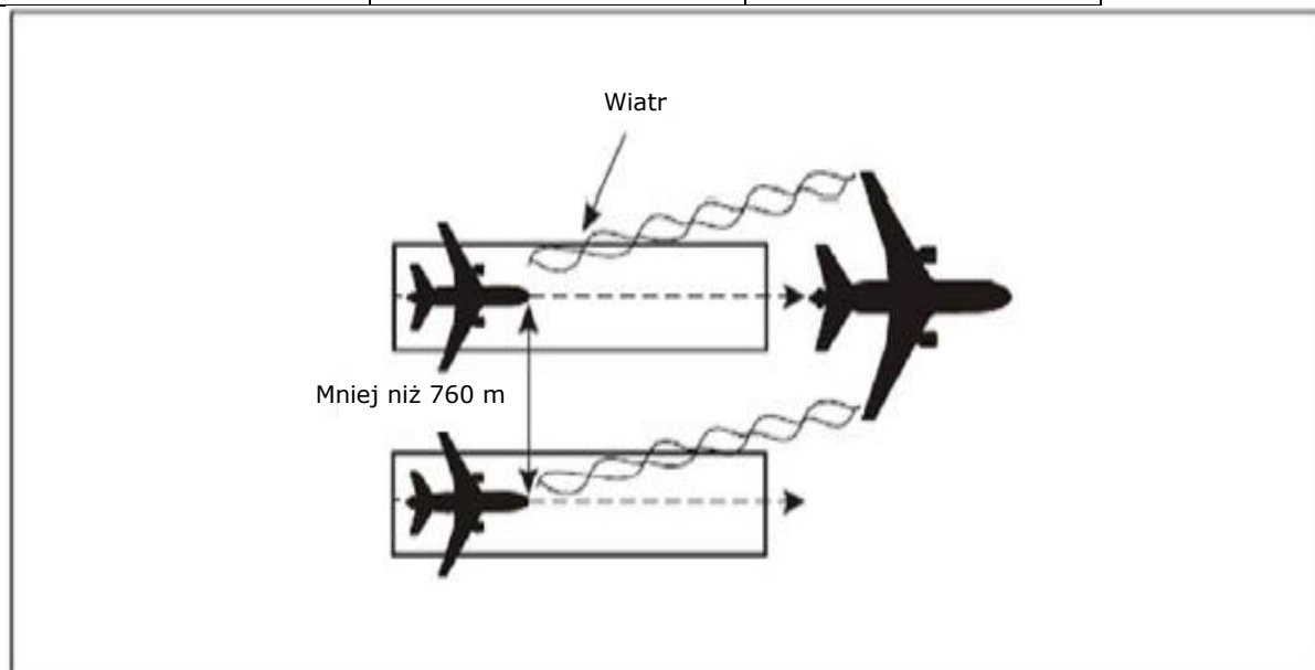
Rysunek 5-42. Separacja za poprzedzającym statkiem powietrznym w warunkach turbulencji w śladzie aerodynamicznym (patrz pkt 5.8.3.1. lit. a) i b) i pkt 5.8.3.2. lit. a) i b))
