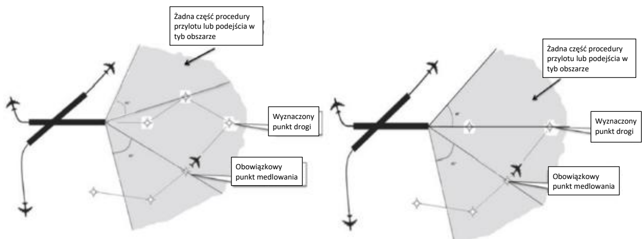
Rysunek 5-41 Przykłady obszaru ochrony przylotowej
