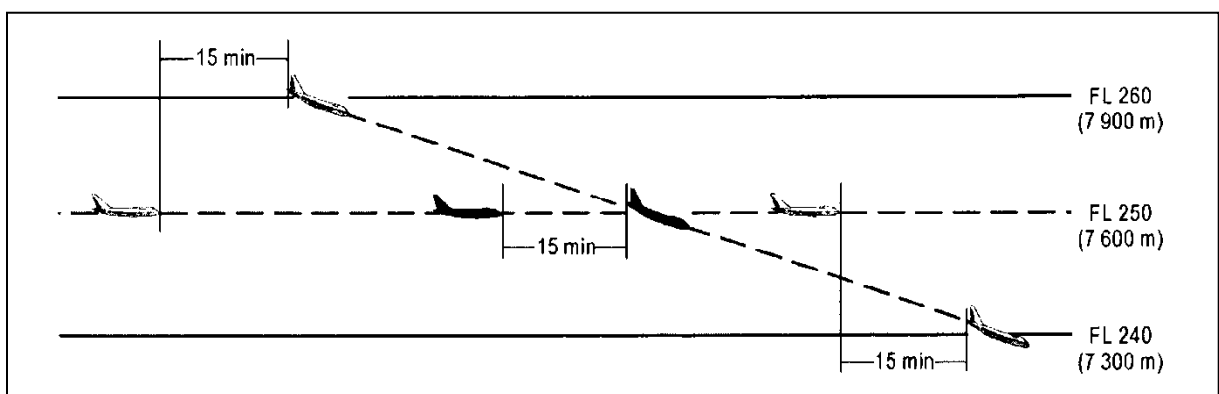
Rysunek 5-16B. Separacja piętnastominutowa między statkami powietrznymi podczas zniżania i na tej samej linii drogi (patrz pkt 5.4.2.2.1 lit. a))
