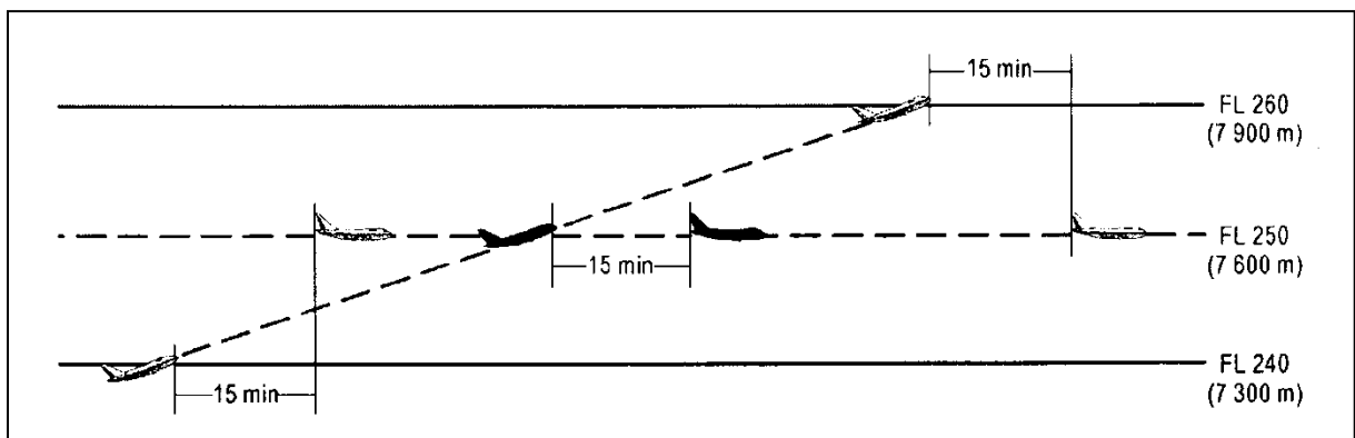
Rysunek 5-16A. Separacja piętnastominutowa między statkami powietrznymi podczas wznoszenia i na tej samej linii drogi (patrz pkt 5.4.2.2.1 lit. a))
