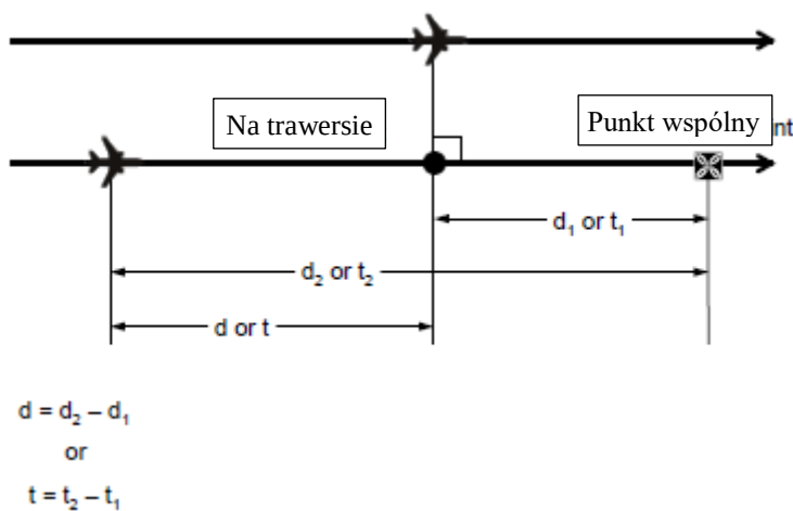
Rysunek 5-34. Obliczanie odległości podłużnej / czasu między statkami powietrznymi – przeciwne strony wspólnego punktu odniesienia (patrz 5.4.2.9.5 b))
