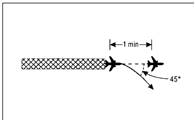
Rysunek 5-37. Separacja jednoczynowa między odlatującymi statkami powietrznymi z kątami drogi różniącymi się nie mniej niż 45^\circ (patrz pkt 5.6.1.)
