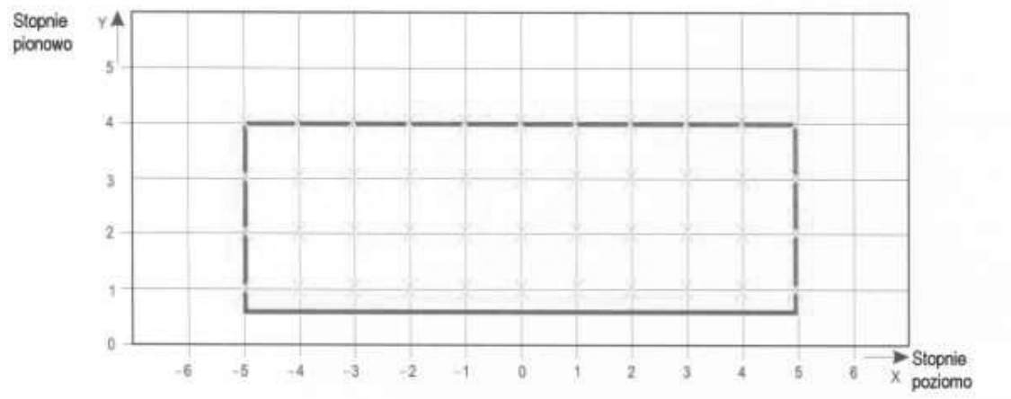
Rysunek A2-21. Punkty siatki służące do obliczeń średniej intensywności światła osi drogi kołowania oraz poprzeczek zatrzymania
