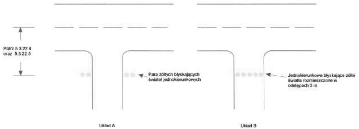
Rysunek 5-28. Światła ochronne drogi startowej
