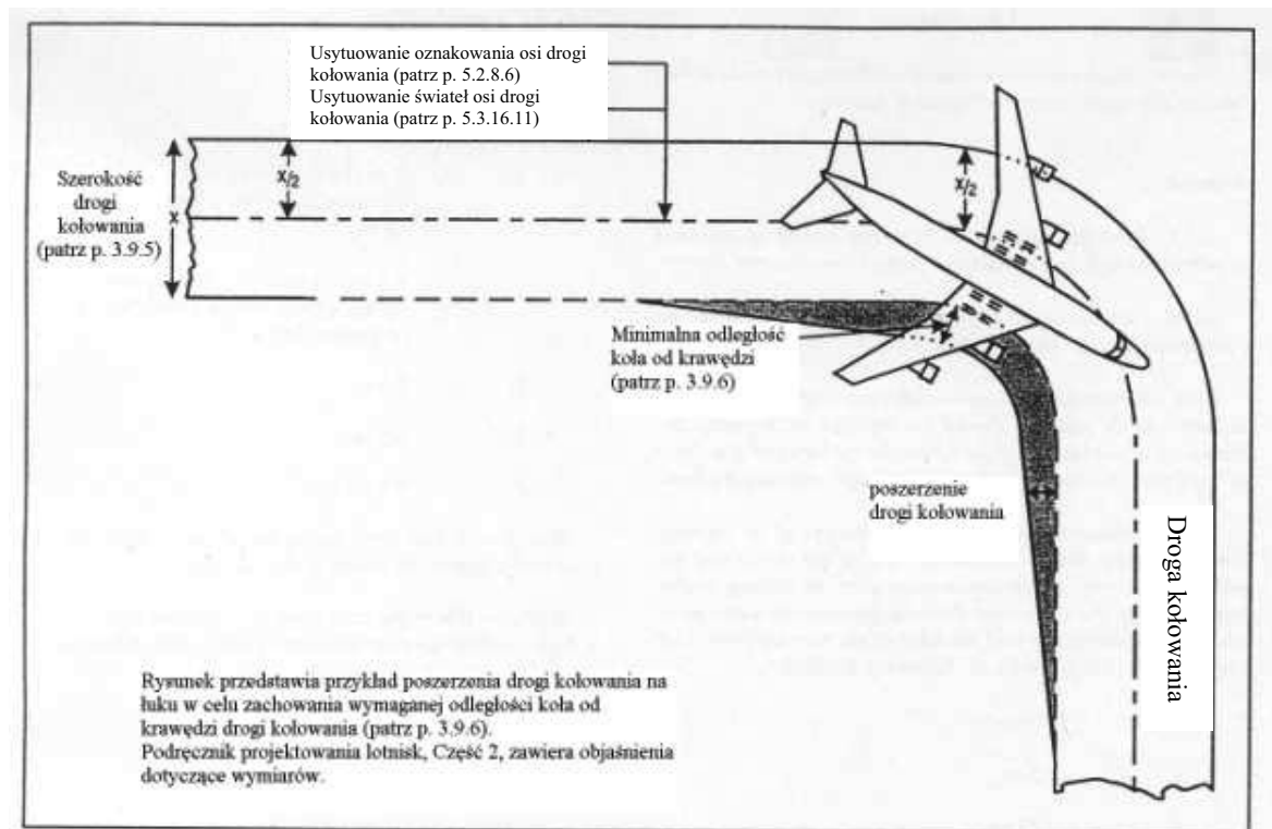
Rysunek 3-2. Łuk drogi kołowania
