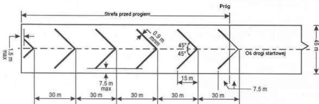
Rysunek 7-2. Oznakowanie powierzchni przed progiem
